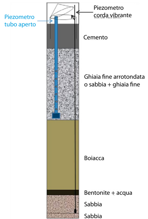
Colonna piezometrica tipo
